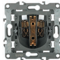
Контактная группа розетки регулярного ассортимента
